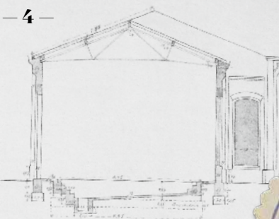
Querschnitt.
