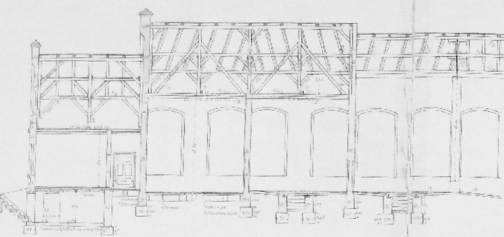
Längsschnitt.
